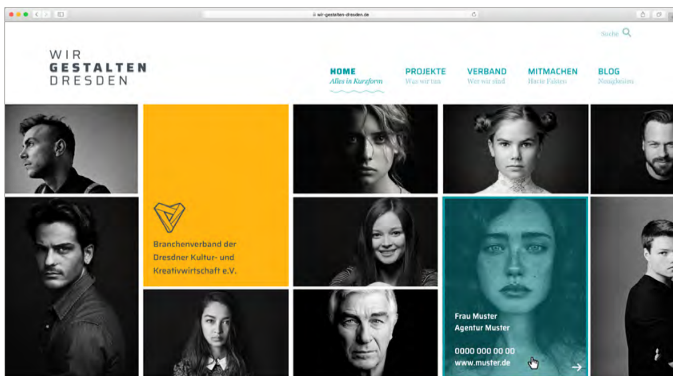
WGD-Startseite Header
